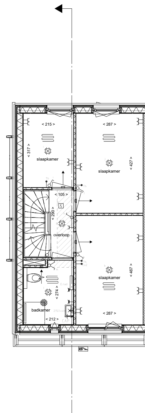
eerste verdieping
