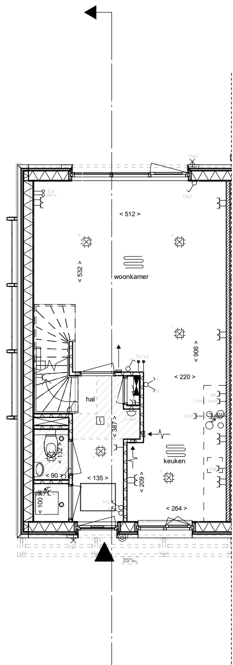
begane grond
